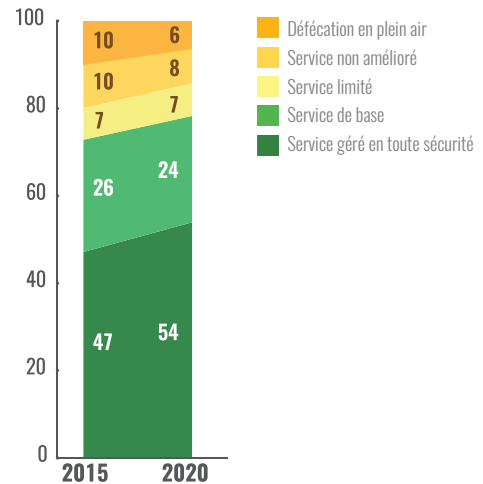
Figure 4 21 : Couverture mondiale des services d'assainissement, 2015-2020 (en %)
