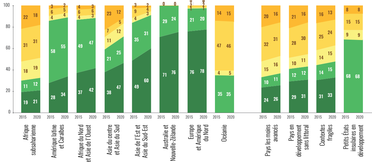
Figure 5 24 : Couverture régionale des services d'assainissement, 2015-2020 (en %)
